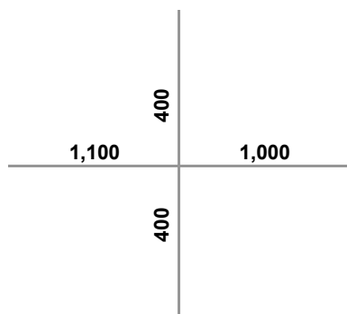
2023 Existing 24-hr. Count (vpd)
